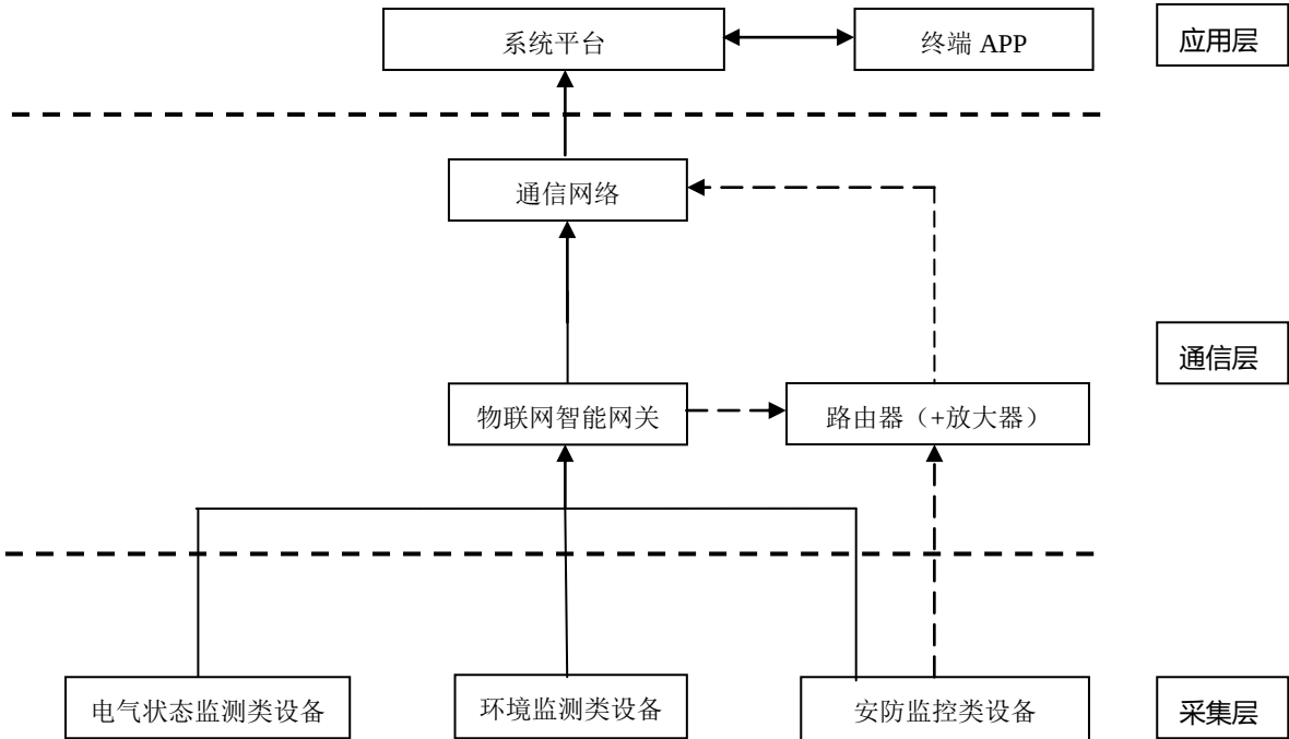
图1 智能配电站系统结构示意图
